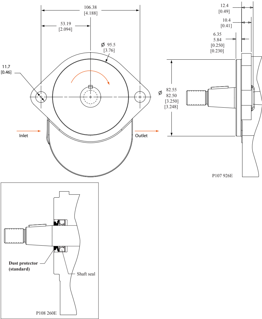
SAE-A 2-bolt flange (AA)
